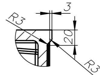
SZCZEGÓŁ C 1 : 3
